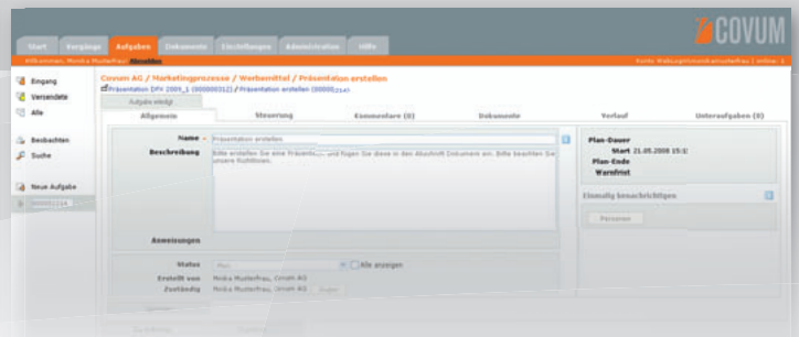
Aufgabenansicht
